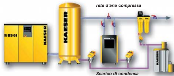
Trattamento dell'aria compressa (filtri, trattamento della condensa, essiccatori ad adsorbimento, colonne ad adsorbimento a carbone attivo)
